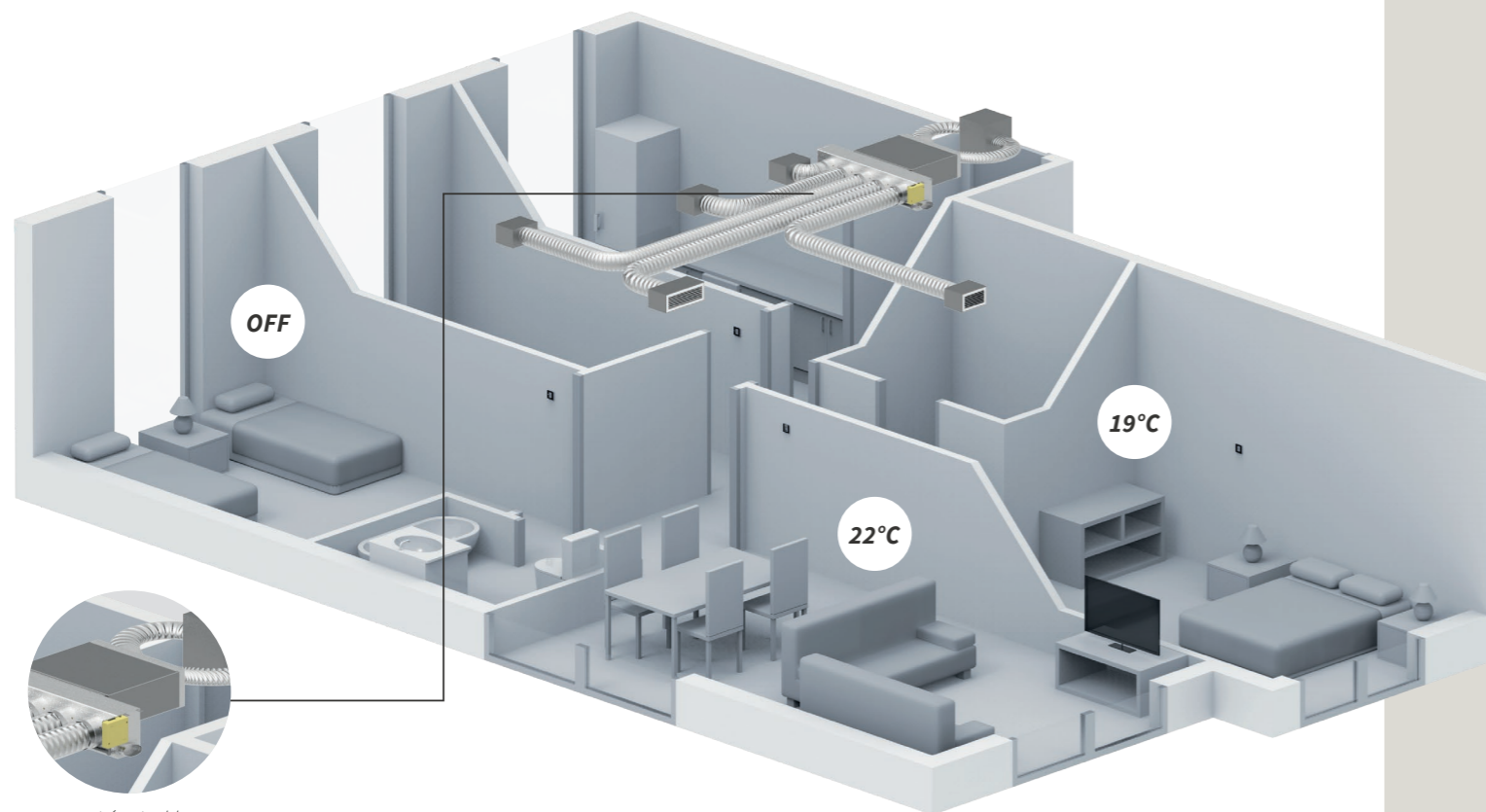
Unité gainable
